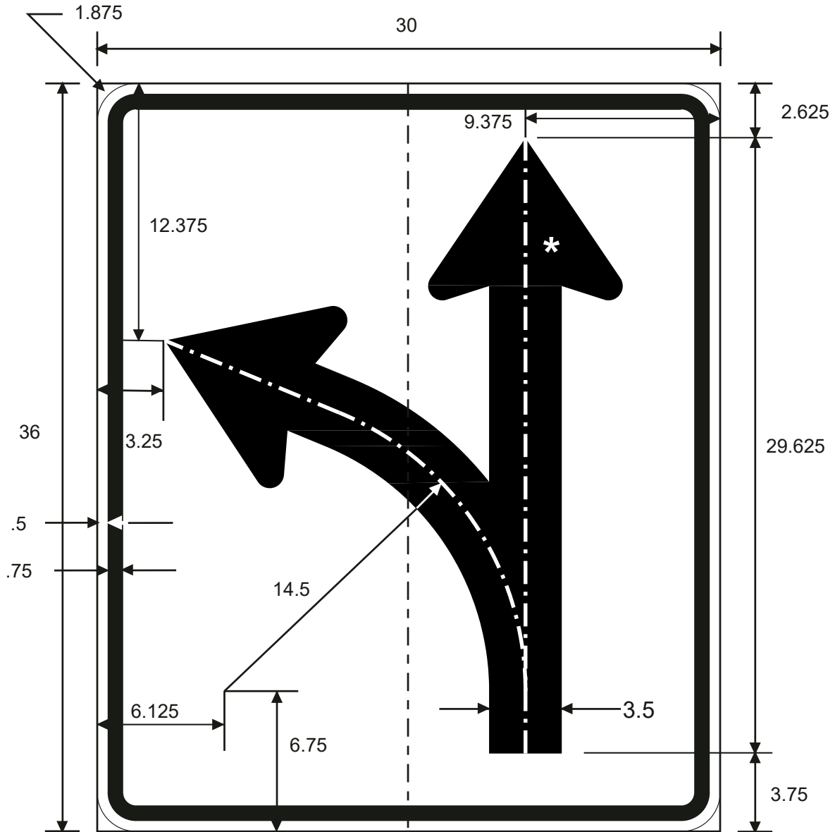
R3-6L Optional Lane Use Arrows
